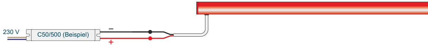
Anschlussbeispiel: Ein LED-Rohr in Reihenschaltung
