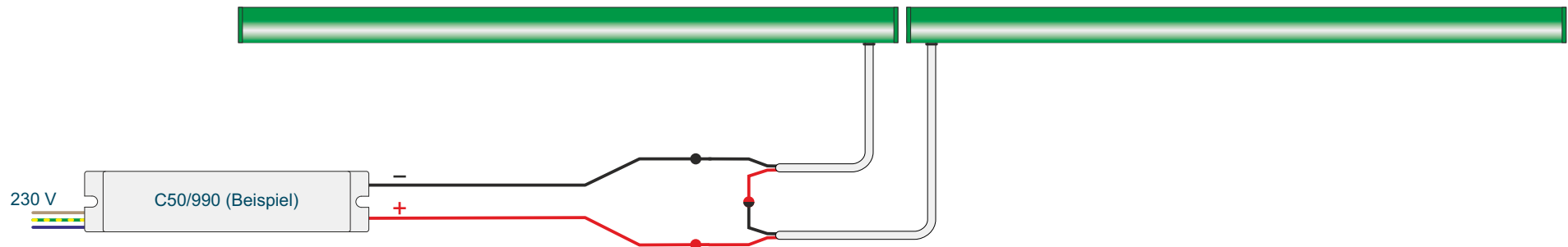
Anschlussbeispiel: Zwei LED-Rohre in Reihenschaltung
