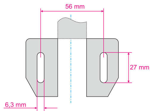
Bohrskizze
