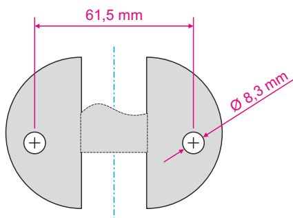
Bohrskizze
