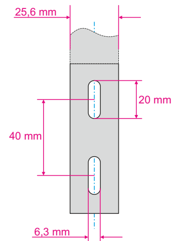
Bohrskizze
